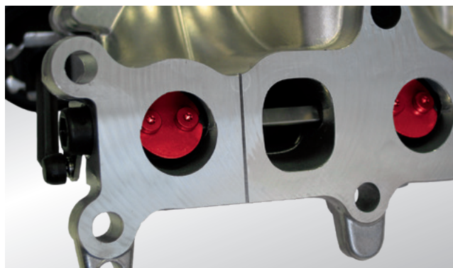
Rys. 2: Po dwa kanały do jednego cylindra: klapę zawirowującą (zaznaczone na czerwono) w rurze dolotowej Pierburg, np. w Oplu Astra J 1.7 CDTi
